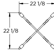
Bottom view counter height Vue de dessous hauteur comptoir
