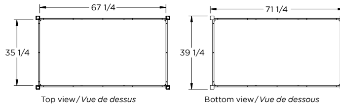
Top view / Vue de dessus
