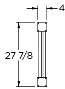
Top view / Vue de dessus
